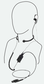
EM-01-581 咽喉マイク & イヤホン ※高騒音下の使用に対応
